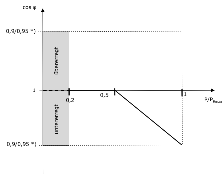
Bild 1: Standard-Kennlinie für \cos \varphi (P) nach VDE-AR-N 4105: 2011-08
