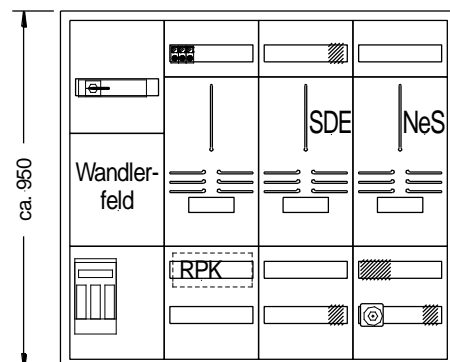
Biogas-BHKW > 100 kW
